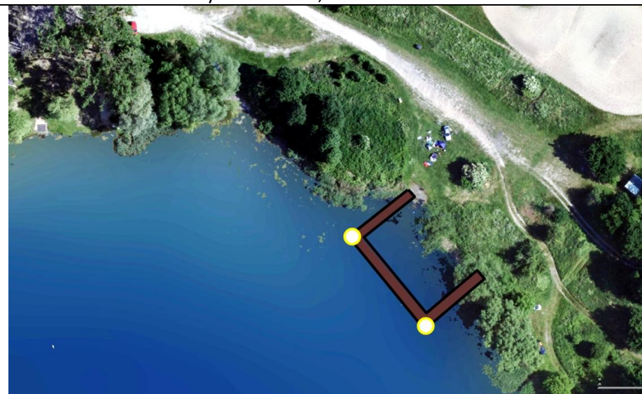
Ryc. 4. Lokalizacja pomostu na terenie Osiedla Kiekrz (posadowienie)
